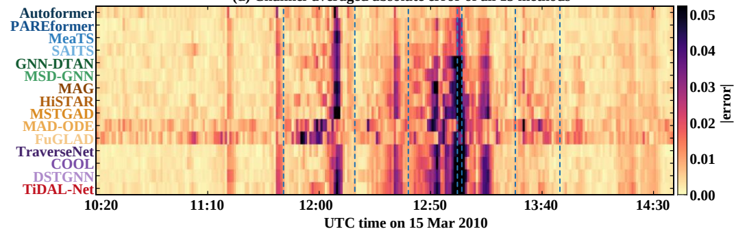
(d) Channel-averaged absolute error of all 15 methods
